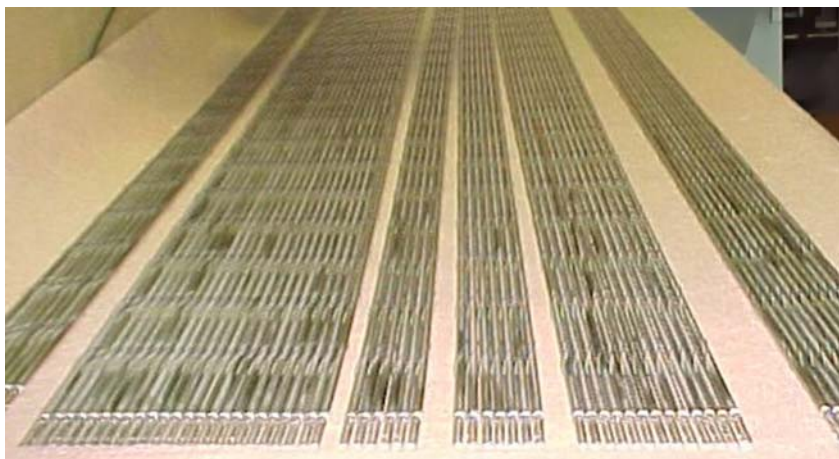
Рис. 3.32. Внешний вид твэлов (а) для гибридной активной зоны реактора БН-800 и их маркировка (б)
